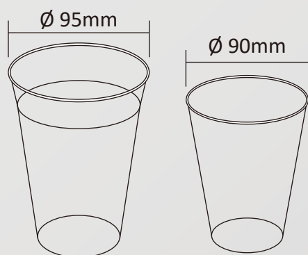
公版規格適用Ø95mm PP膠杯及 Ø90mm PE紙杯。
